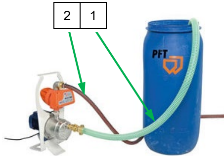
Abb. 5: Druckerhöhungspumpe aufstellen
